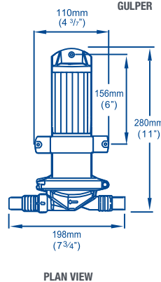
GULPER
